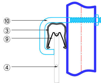
⊙ 주립 상세도 SCALE : NONE
