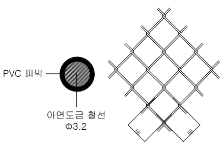
PVC 코팅망 상세도 SCALE : NONE
