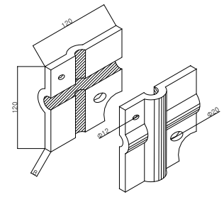
교차조립구 상세도 SCALE : NONE
