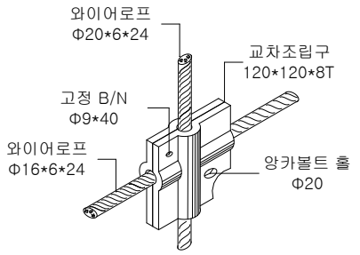
교차조립구 연결 상세도 SCALE : NONE
