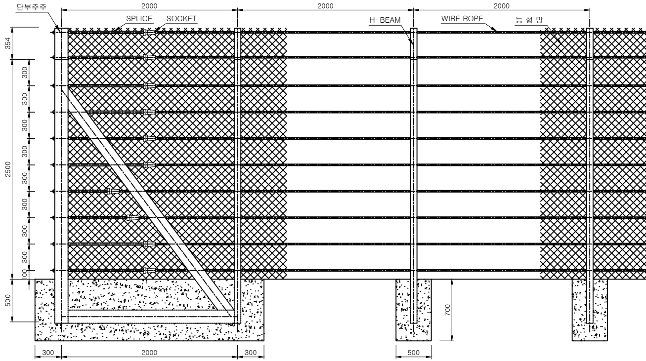
설치 전개도 Scale = 1: none
