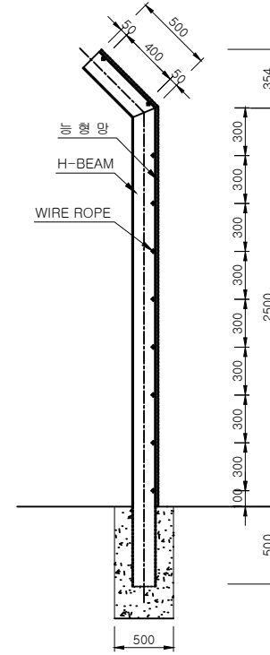
주주 부분 상세도 Scale = 1: none
