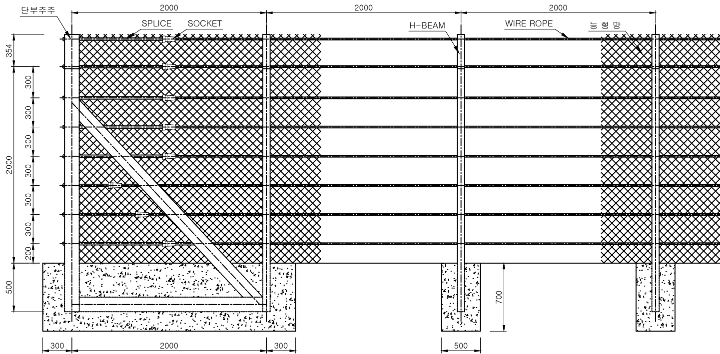
설치 전개도 Scale = 1: none
