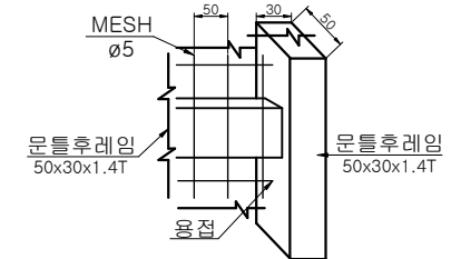
MESH 조립도
