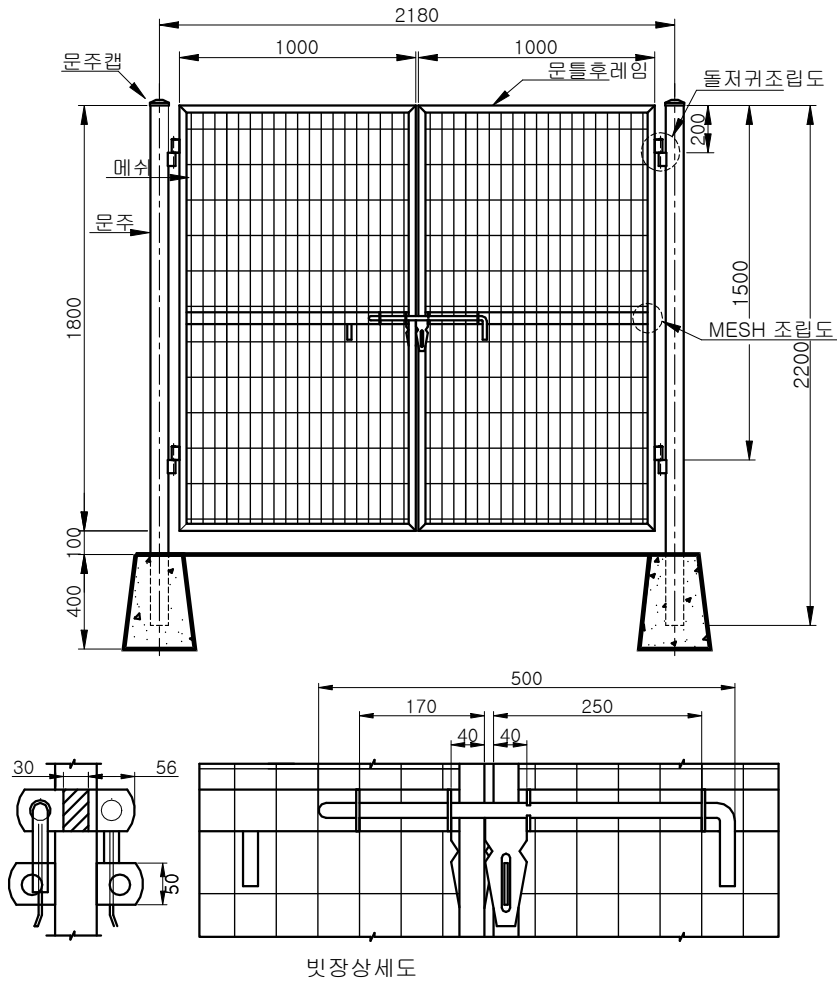
입면도
