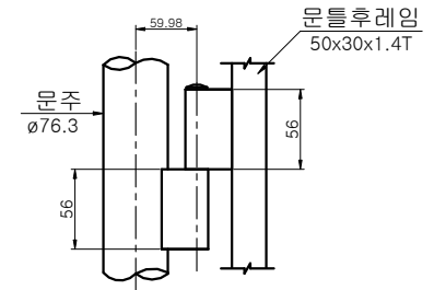
돌저귀 조립도
