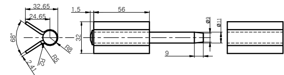
돌저귀 부품도
