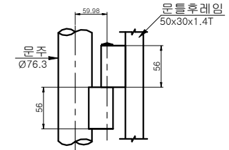
돌저귀 조립도
