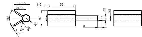
돌저귀 부품도
