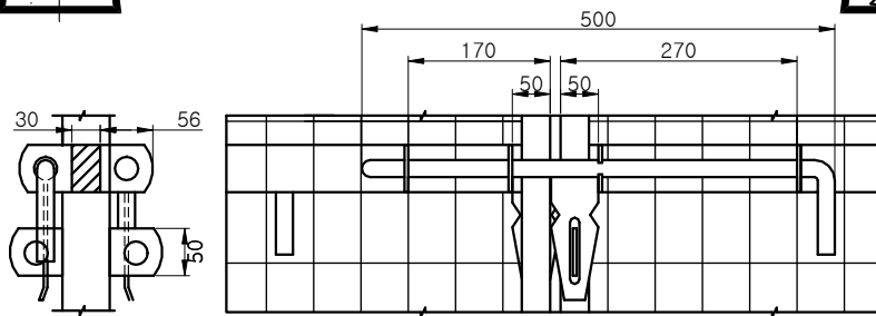
빗장상세도
