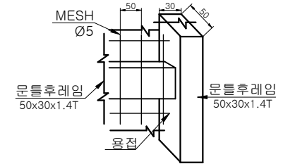
MESH 조립도
