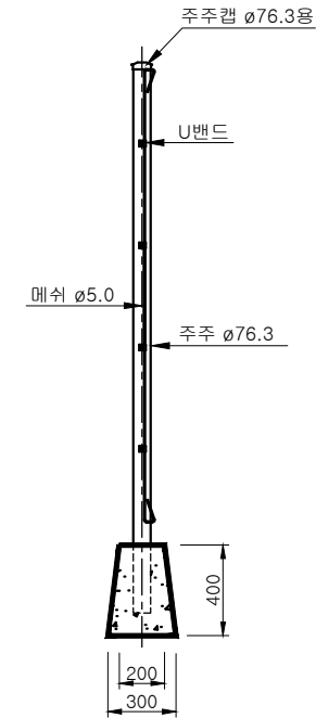
○ 주주 부분 상세도 SCALE : 1 / NO
