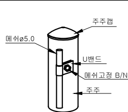
메쉬 U밴드 조립도
