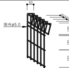
메쉬철선 배열도
