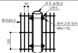
메쉬 주주 조립도
