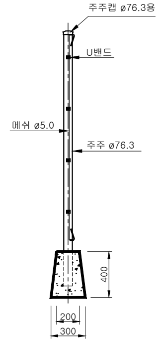
○ 주주 부분 상세도 SCALE : 1 / NO
