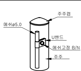
메쉬 U밴드 조립도
