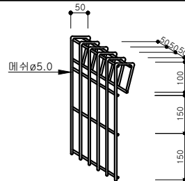
메쉬철선 배열도
